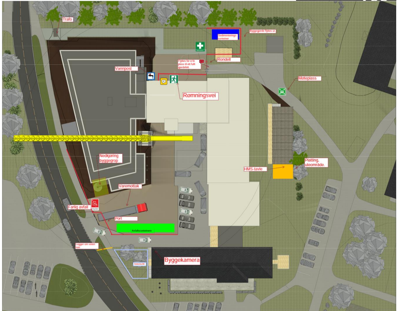
Riggplan 1.etappe (Grunnarbeider)
